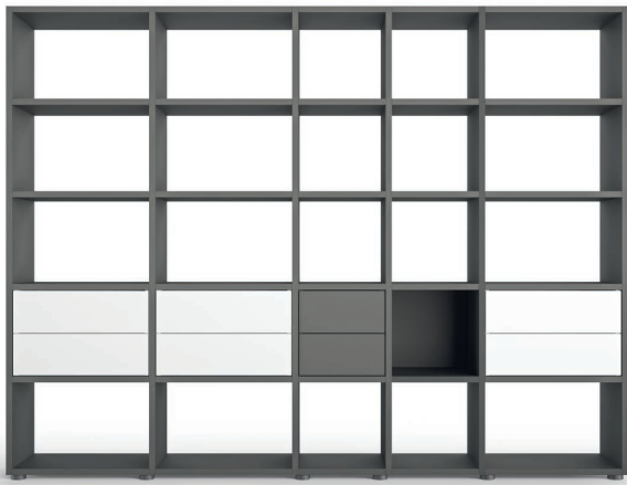
B 250 cm, H 190,3 cm (5 OH), T 36 cm 4 x Schubläden/1 x Rückwand
